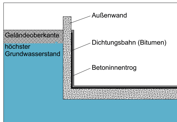
„Schwarze Wanne“ Innendichtung
