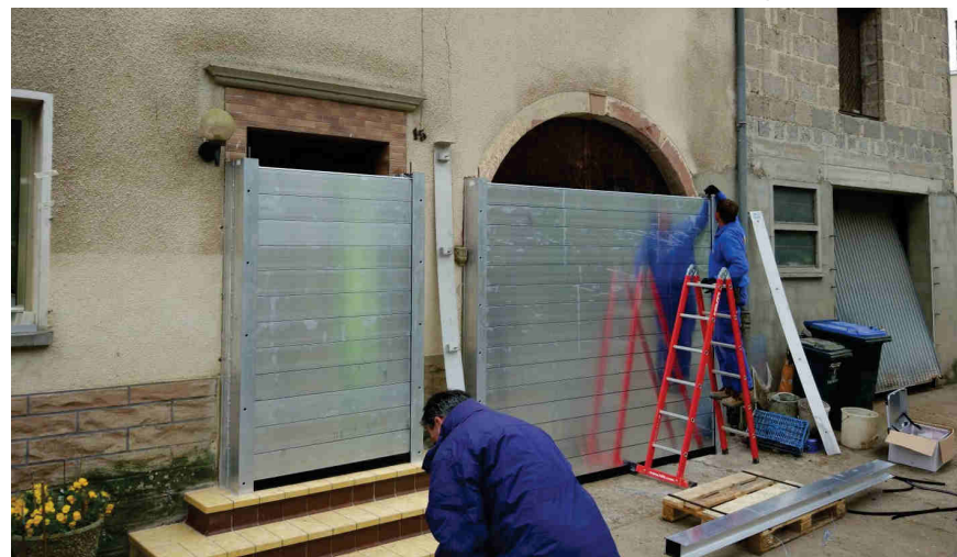
temporäres Dammbalkensystem
